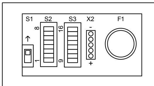
Рис 1. Отсек переключателей.
