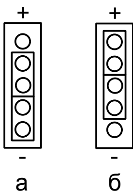
Рис. 2. Установка полярности счётных импульсов: а - отрицательная, б - положительная.
